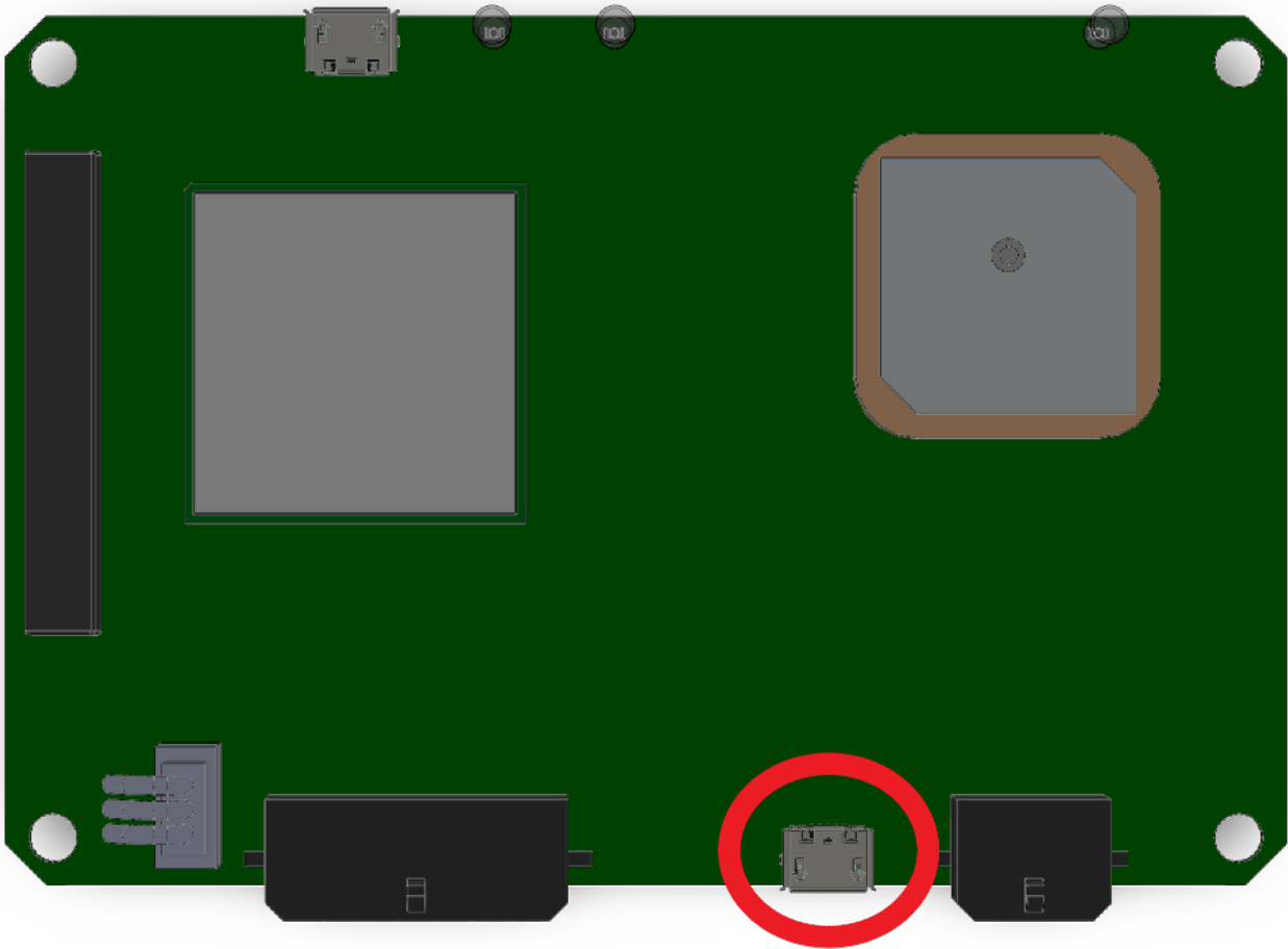
Рис. 12 Расположение microUSB-разъёма.
