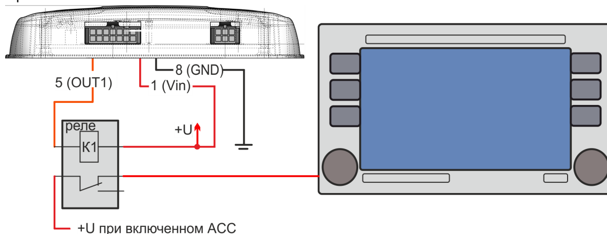
Рис. 15 Схема подключения автомагнитолы.
