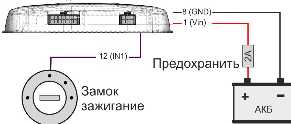
Рис. 14 Схема подключения.
