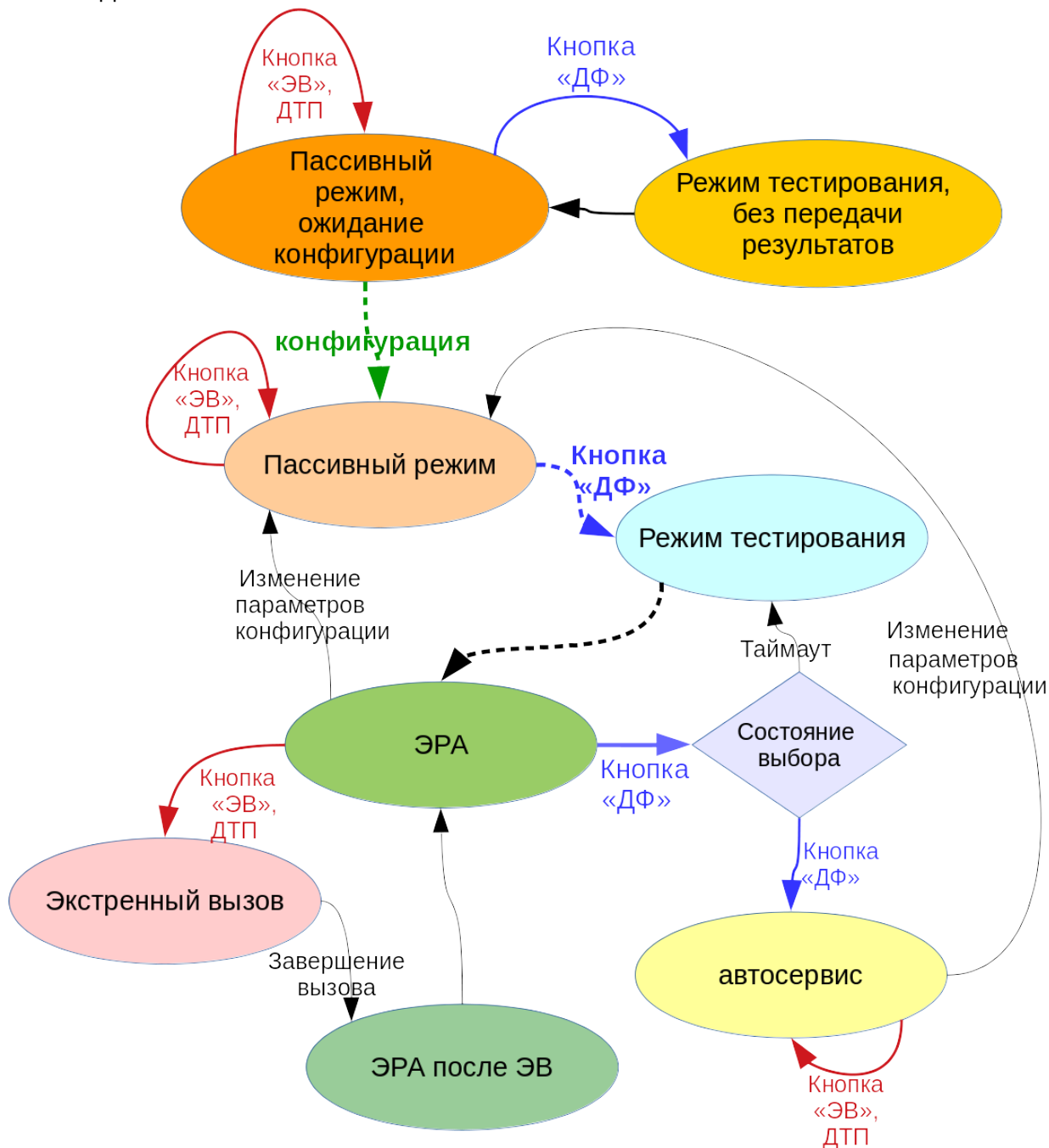
Рис. 9 Диаграмма состояний.
